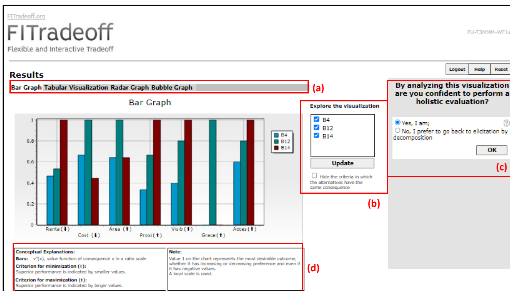
Figura 26 – Tela de Avaliação Holística para a problemática de escolha
