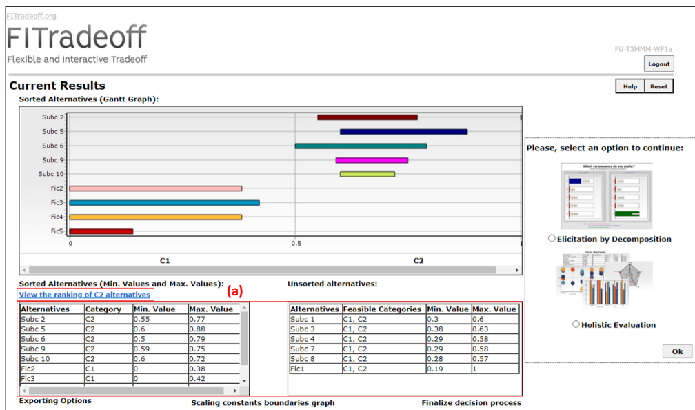
Figura 39 – Resultados parciais para a problemática de classificação
