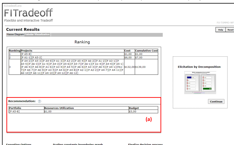
Figura 40 – Resultados parciais para a problemática de portfólio
