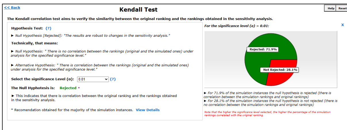
Figura 49 – Tela do teste de Kendall na análise de sensibilidade para a problemática de ordenação com relatório do coeficiente de Kendall
