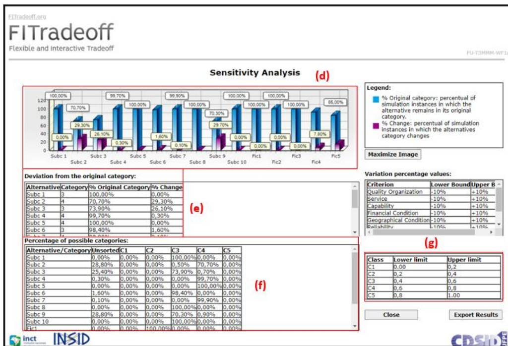
Figura 50 – Tela da Análise de Sensibilidade para a problemática de classificação
