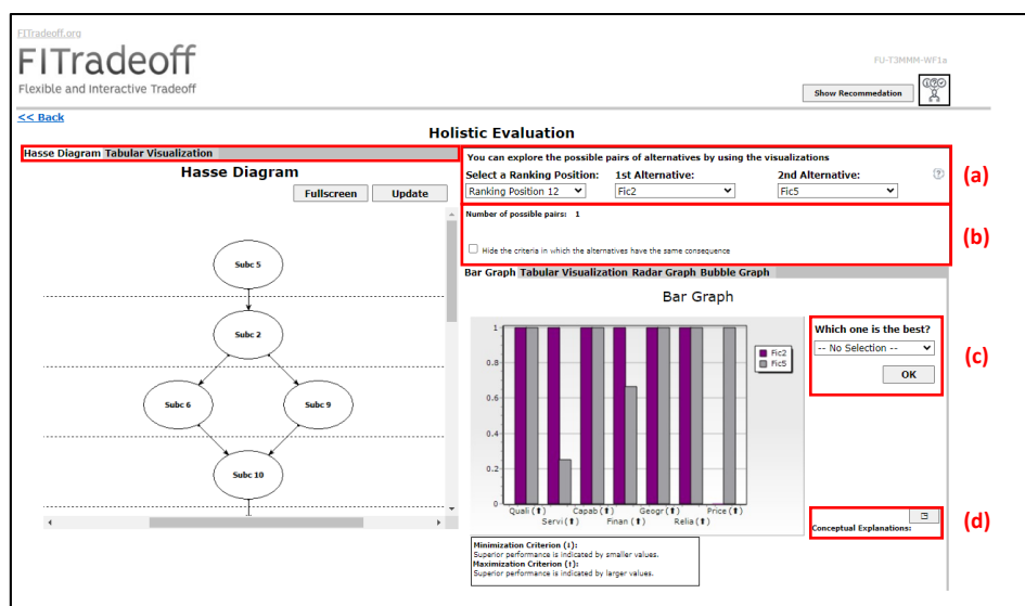
Figura 28 – Tela de Avaliação Holística para a problemática de ordenação
