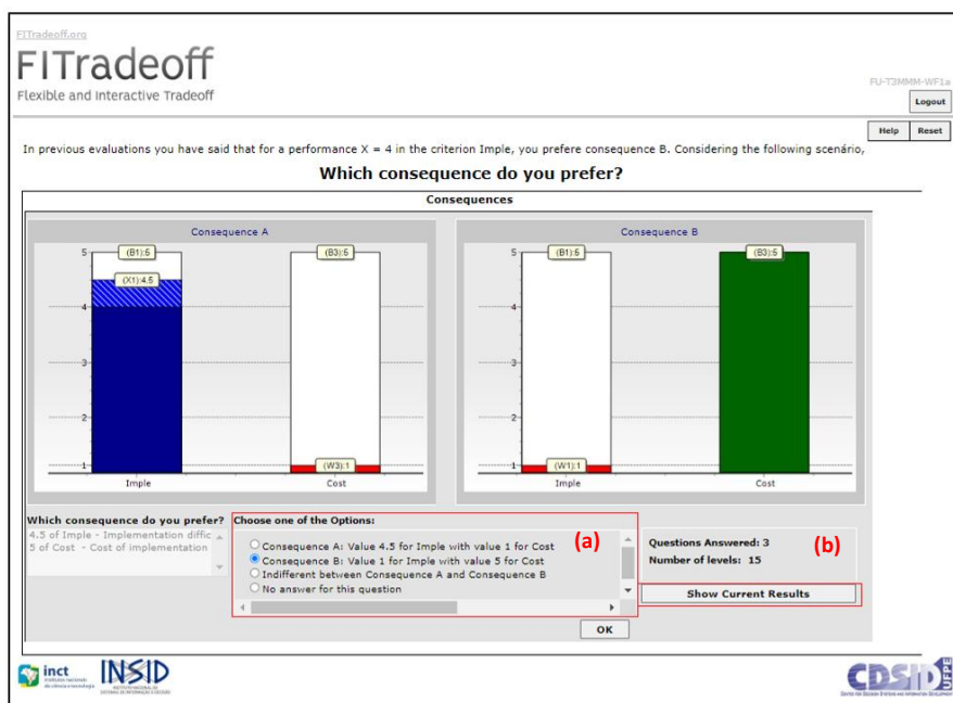
Figura 25 – Caso de elicitación por níveis intermediários
