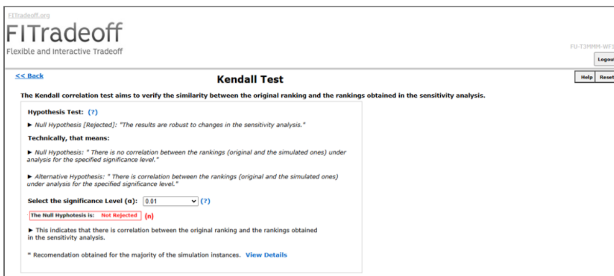
Figura 49 – Tela do teste de Kendall na análise de sensibilidade para a problemática de ordenação com relatório do coeficiente de Kendall
